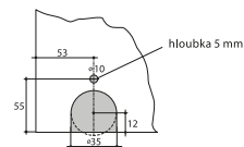
schéma montáže
