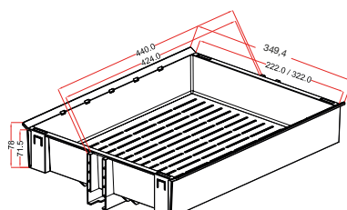
korpus 400 mm
