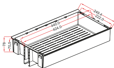
korpus 300 mm
