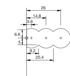
opracování korpusu
