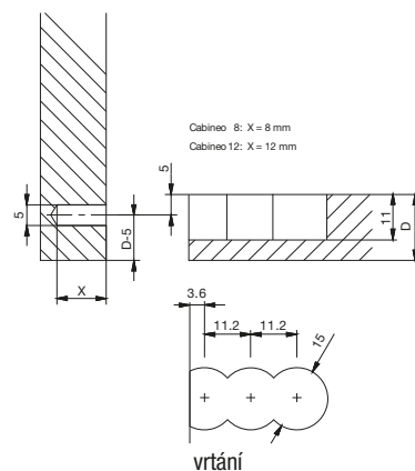
vrtání
