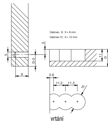
vrtání
